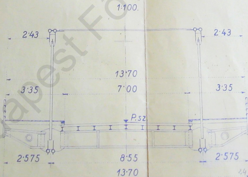
VASSZERKEZETI ÁTHIDALÁS METSZETE.
