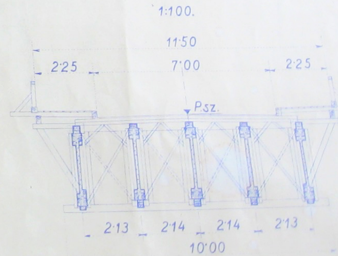
SZEGEZETT FASZERKEZETI ÁTHIDALÁS METSZETE.
