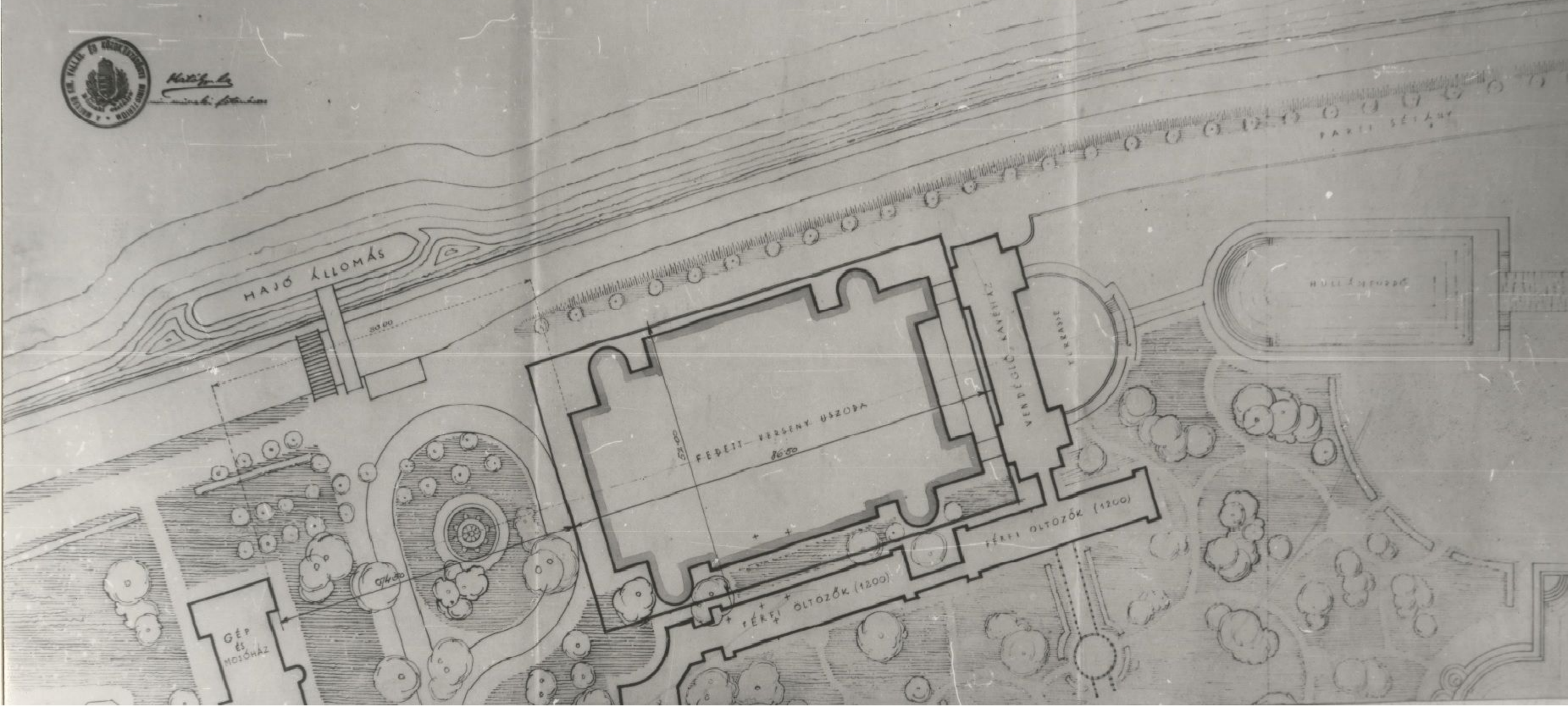
SZT. MARGITSZIGETI FEDETT VERSENYUSZODA ELHELYEZÉSI TERVEZETE TERVEZŐ: HAJÓS ALFRÉD ÉPÍTÉSZMERNŐK
