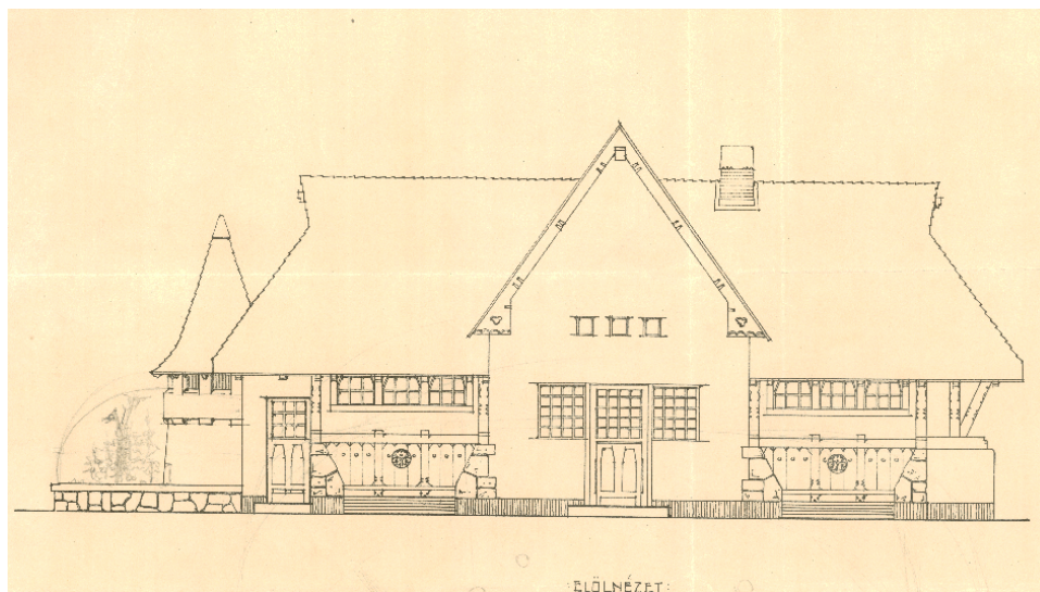
5. kép A kenguruház lehetne egy falusi közintézmény is (BFL XV.d.17.328 KT szor 1/46-1)
