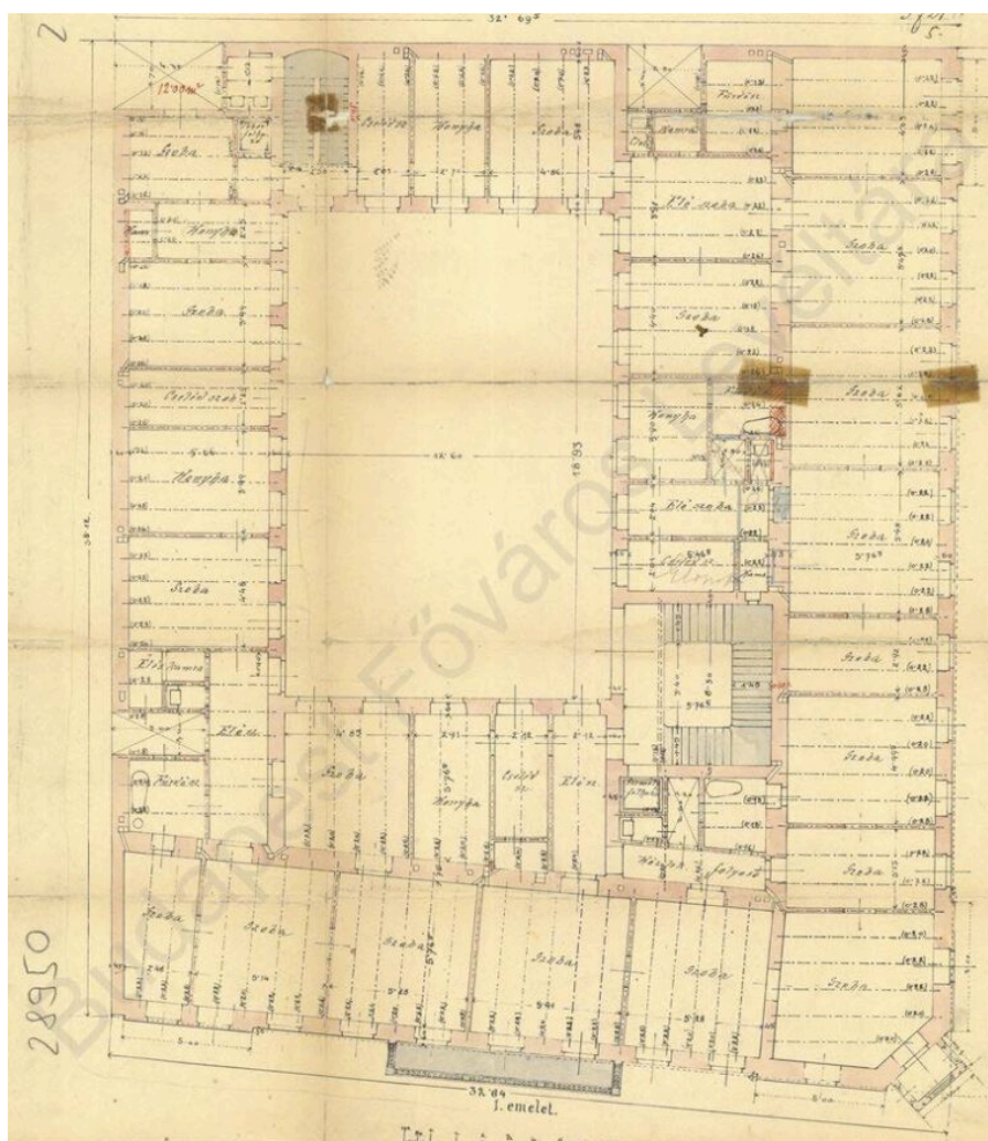
2. kép. A Gyár utca 26. sz. ház I. emeleti alaprajza, 1895. (BFL XV.17.d.329 - 28950 4. f.)
