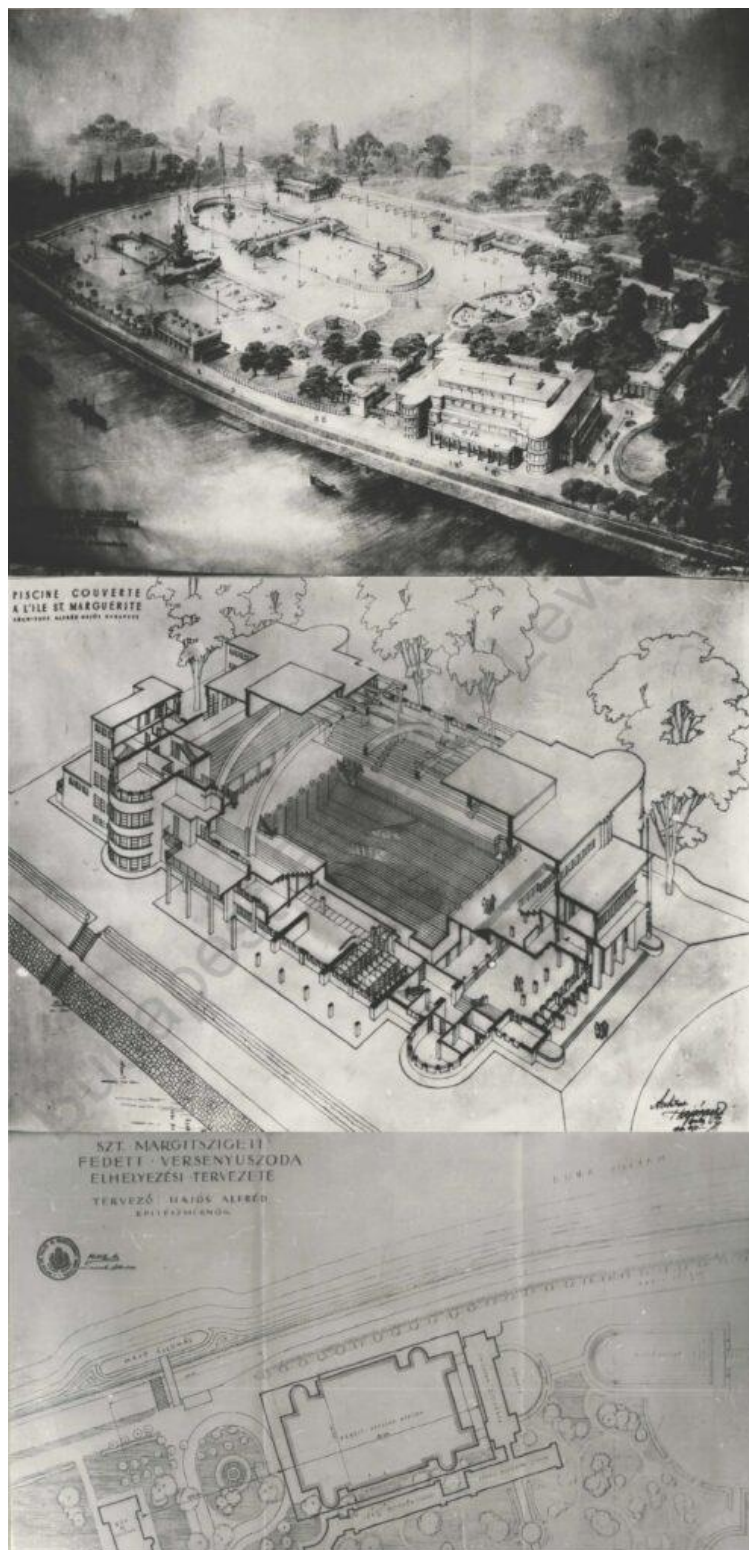
A Nemzeti Sportuszoda elhelyezési vázlata, perspektivikus metszete és elhelyezési terve (BFL XV.17.e.306 3258)
