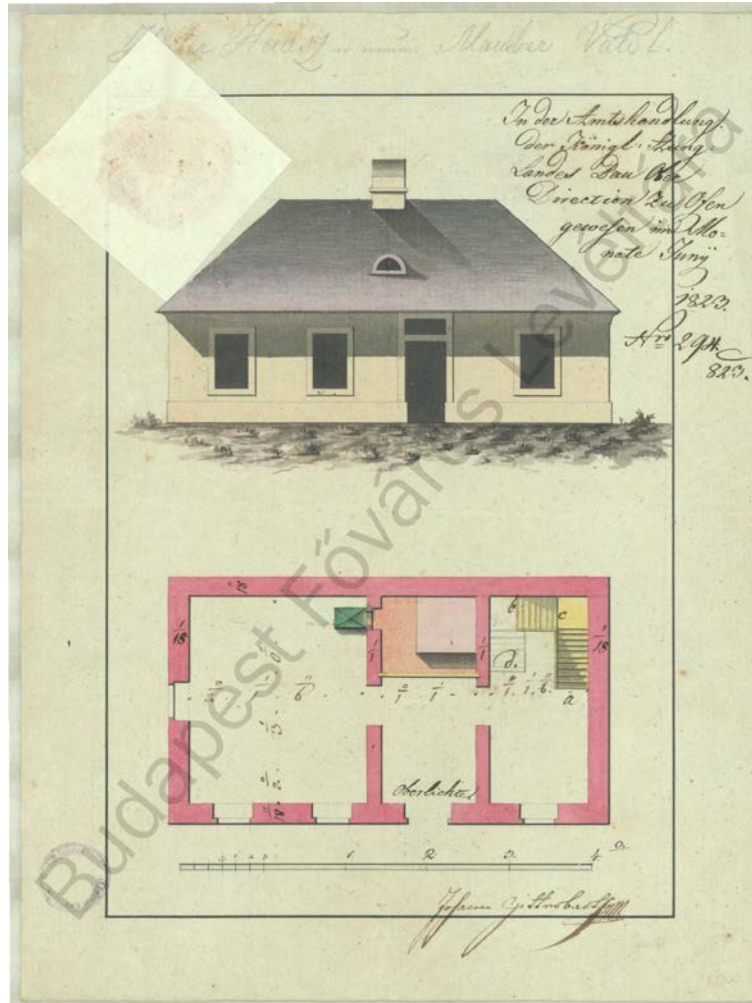
7. kép. Az „új epreskert”-be tervezett, Zitterbarth János szignójával ellátott csőszház terve, 1823. (BFL XV.17.b 314. 15/a.)
