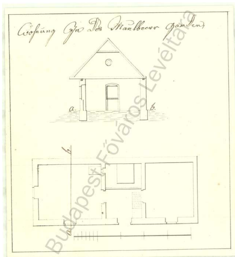
5. kép. A tervezett epreskerti kertész- vagy csőzház terve, 1800 (BFL XV.17.b 314. 13.)
