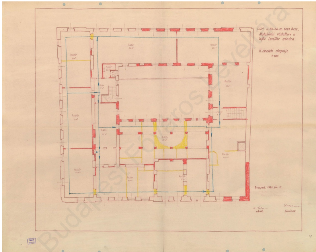
6. kép. Az épület tervezett második szintje. (BFL VIII.3801.a. 27. tétel)
