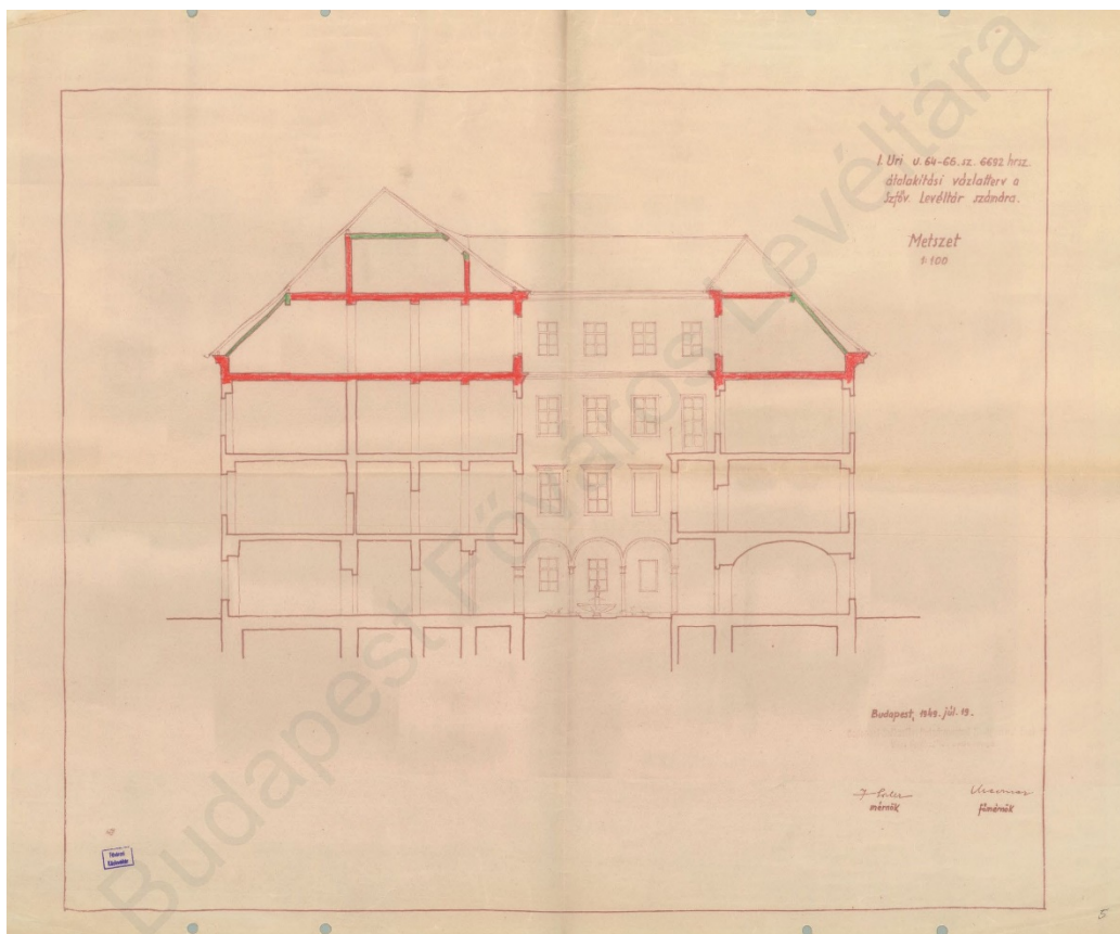
9. kép. Az épület metszet rajza. (BFL VIII.3801.a. 27. tétel)
