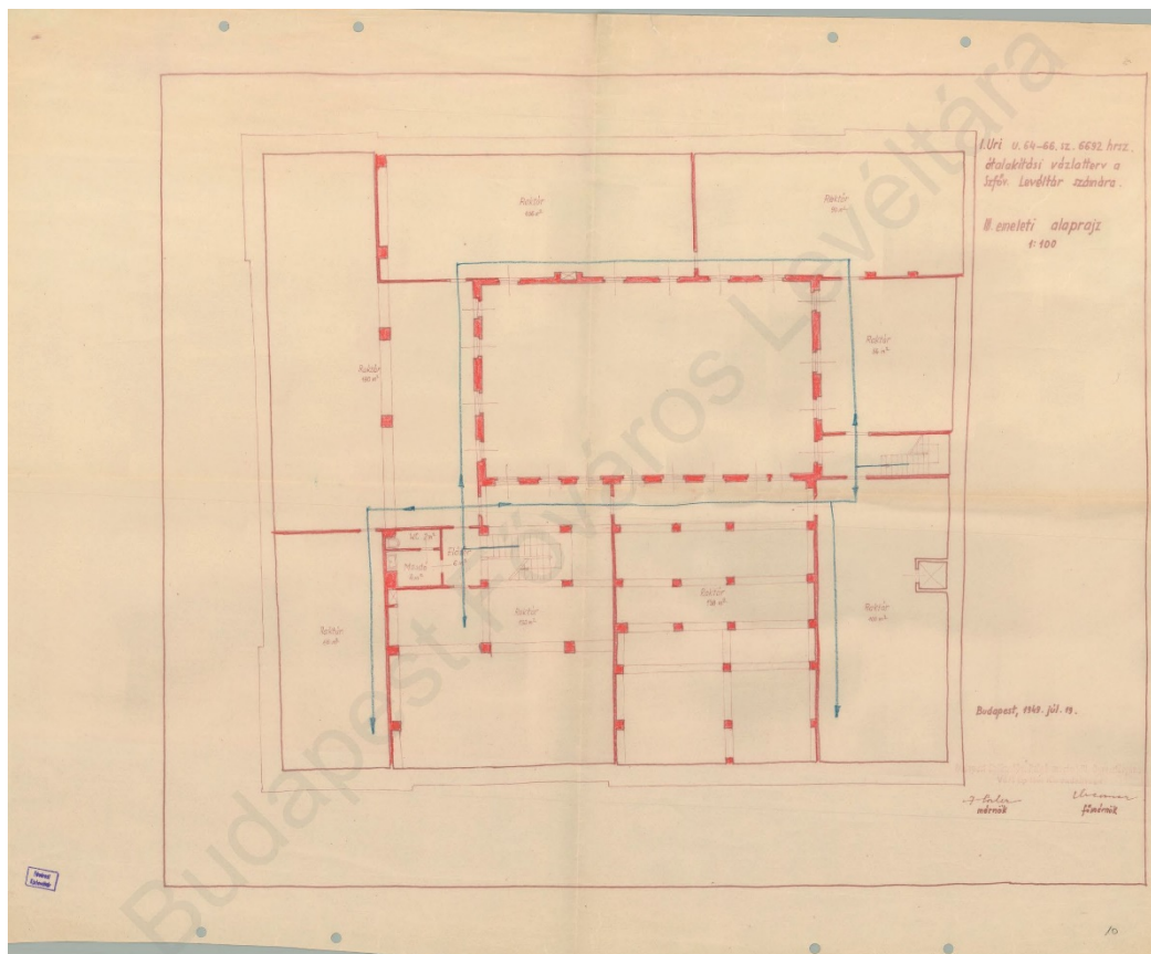
7. kép. A tervezett III. szint. (BFL VIII.3801.a. 27. tétel)
