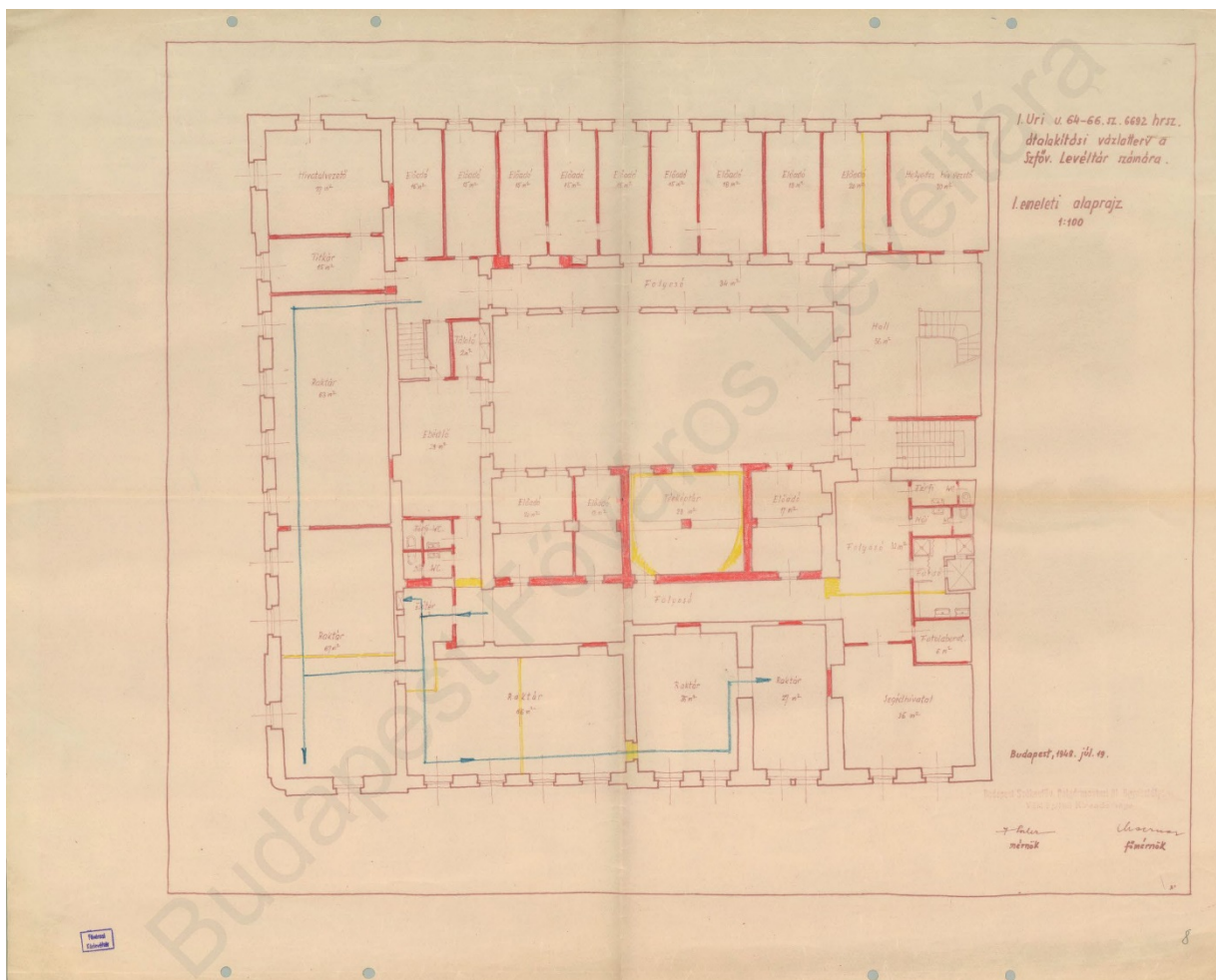
5. kép. Az épület első szintjének tervrajza. (BFL VIII.3801.a. 27. tétel)
