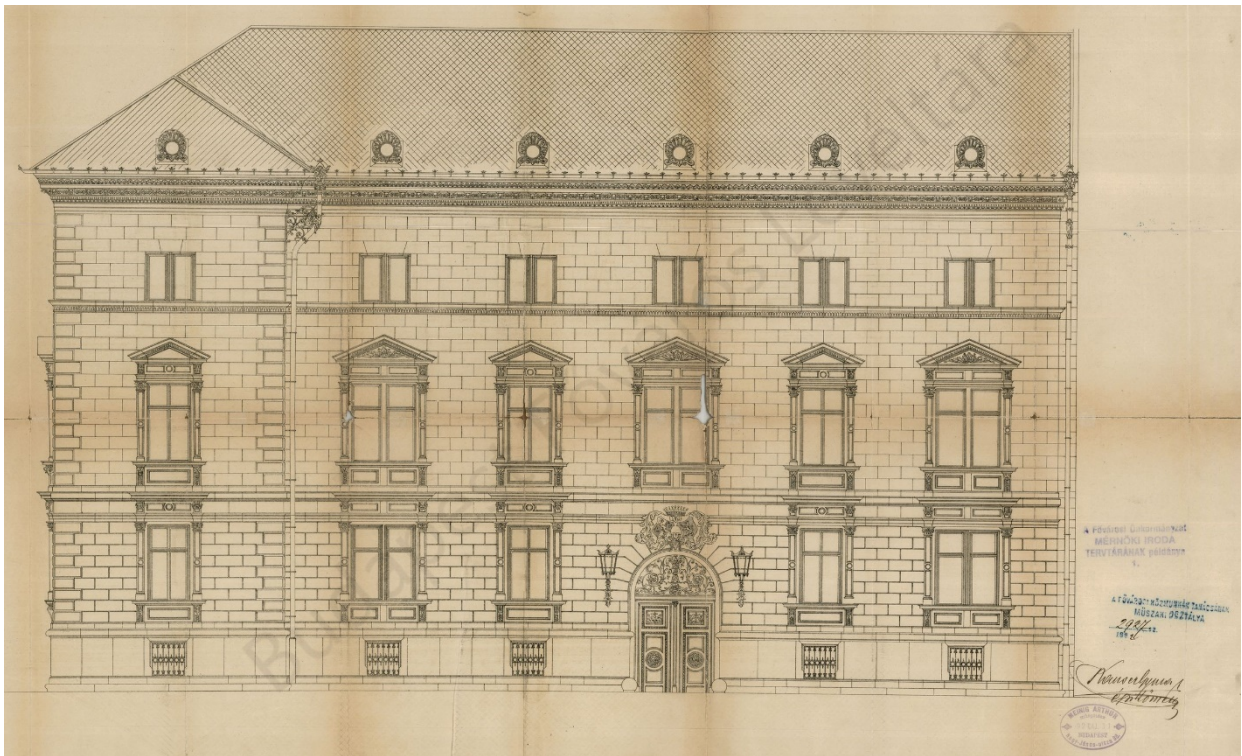
7. kép. A Hunyady-palota homlokzatának terve. (BFL XV.17.d.329. 36534-8)
