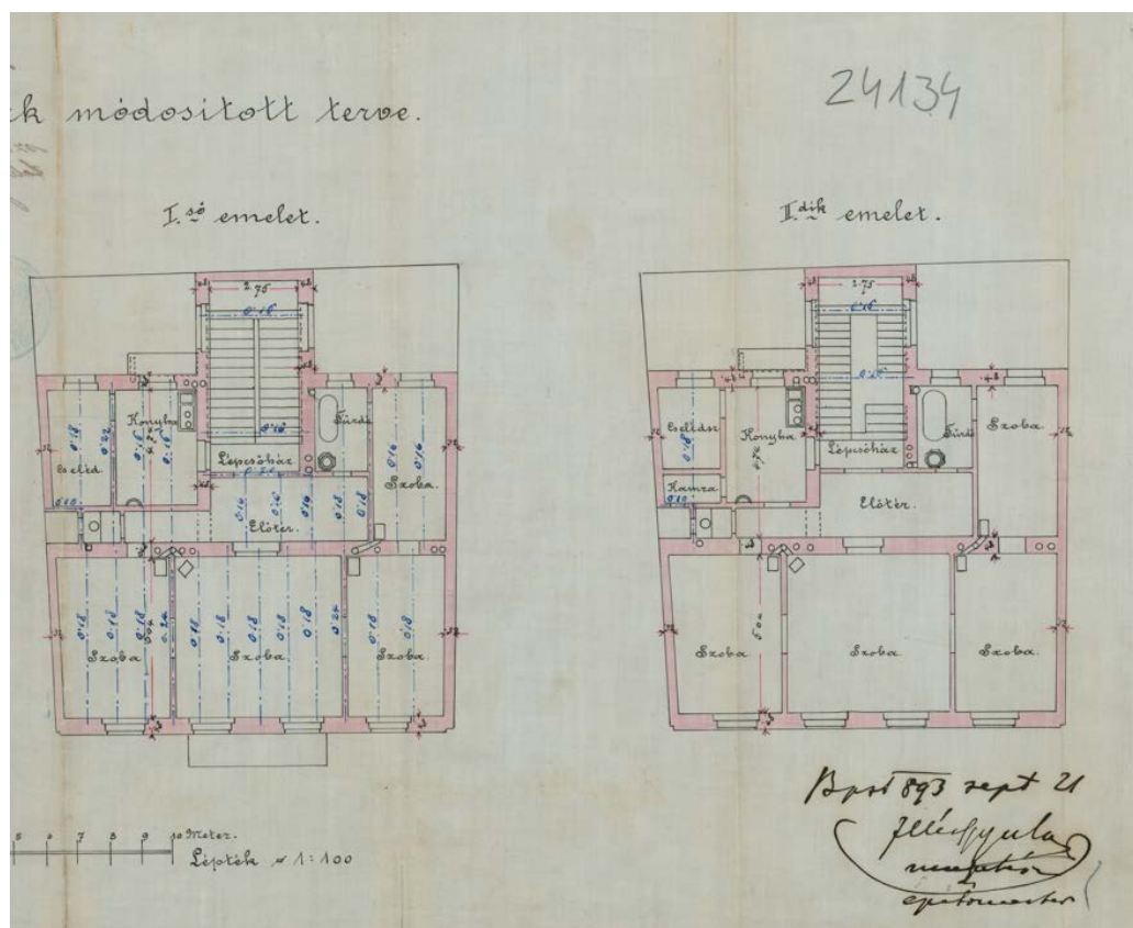
3. kép. A Magyar utca 20. alatti ház első és második emeletének terve. Illés Gyula, 1893. ( BFL XV.17.d.329 24134 , részlet)
